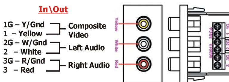
Цоколевка
